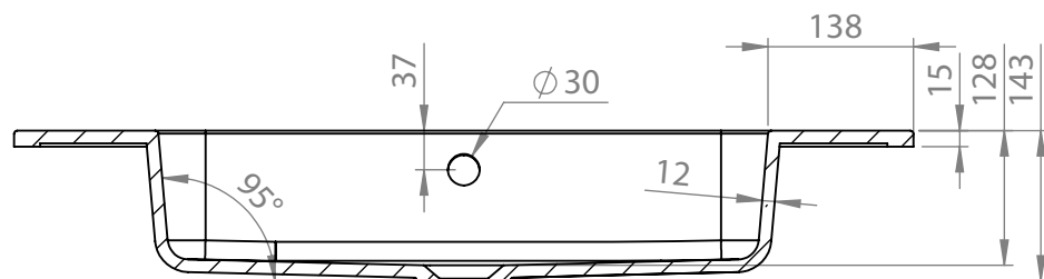
PRZEKRÓJ N-N SKALA 1 : 8
