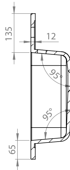
PRZEKRÓJ M-M SKALA 1 : 8
